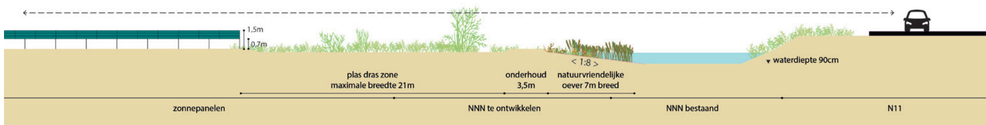
Principedoorsnede 4: nieuwe situatie, zonnepanelen maximaal 1,5m hoog zodat zicht vanaf verhoogde N11 over de panelen heen goed mogelijk is. De nieuwe NNN-zone wordt ingericht met een brede natuurvriendelijke oever en een afgegraven zone van wisselende breedte tussen oever en de panelen. Op bovenstaand profiel is de maximale breedte zichtbaar.
