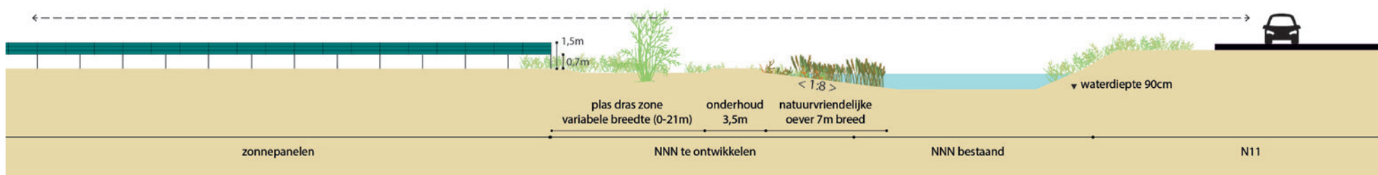
Principedoorsnede 2: nieuwe situatie, zonnepanelen maximaal 1,5m hoog zodat zicht vanaf verhoogde N11 over de panelen heen goed mogelijk is. De nieuwe NNN-zone wordt ingericht met een brede natuurvriendelijke oever en een afgegraven zone van wisselende breedte tussen oever en de panelen.
